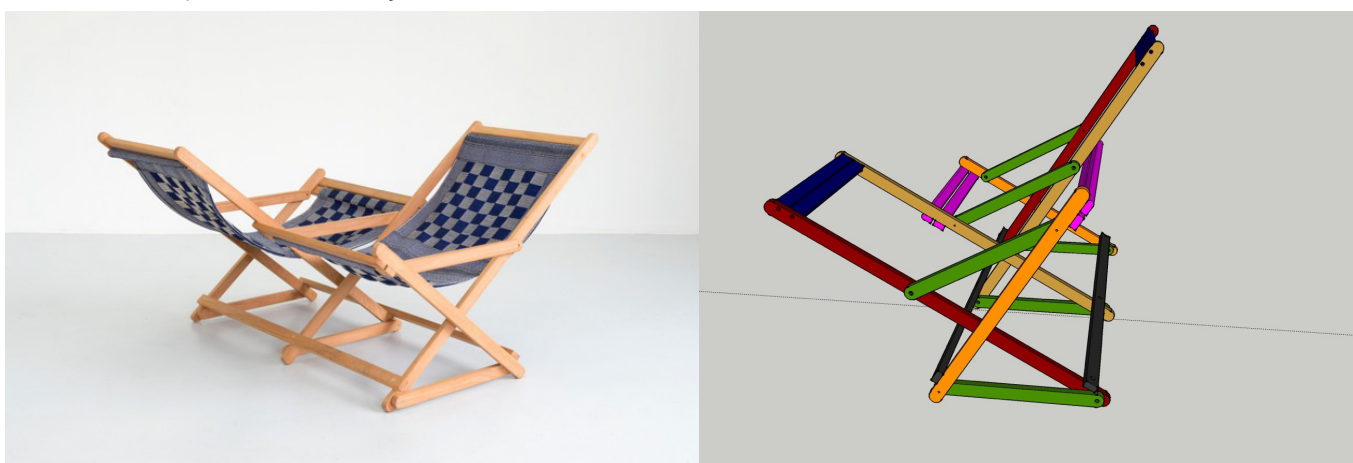
Transat Nord/Sud et modélisation en vue de son amélioration réalisée par un étudiant du LMB
